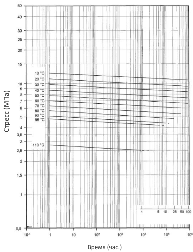
PE-X диаграмма механического сопротивления (EN ISO15875-2)
